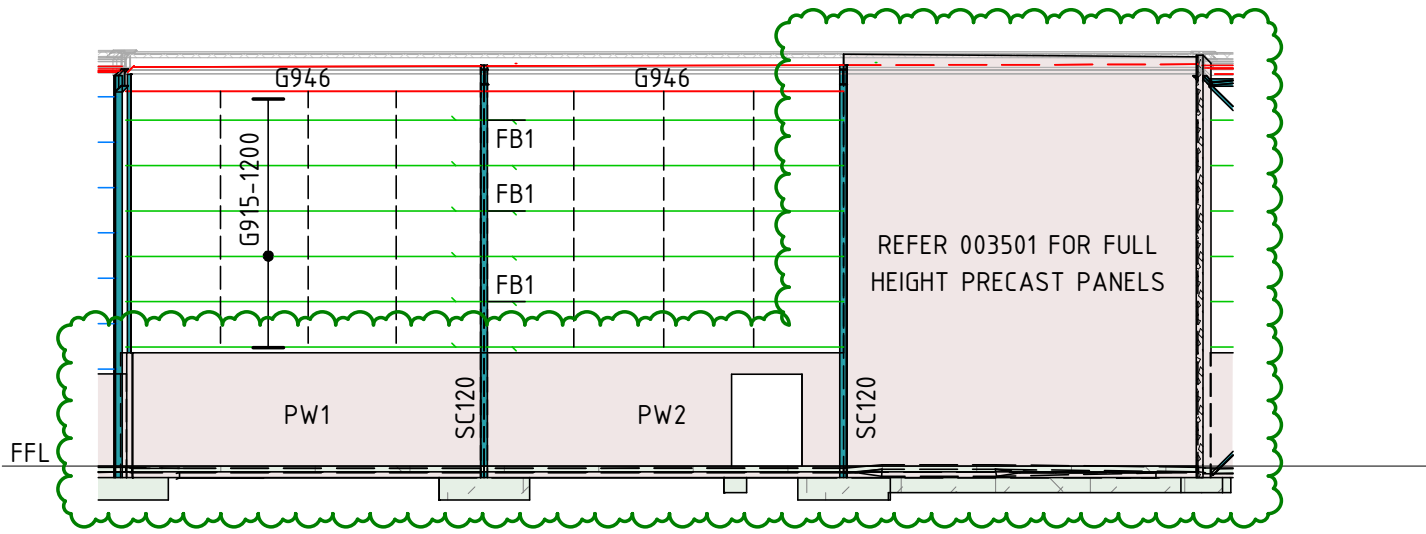
SECTION 1B SCALE 1 : 200
